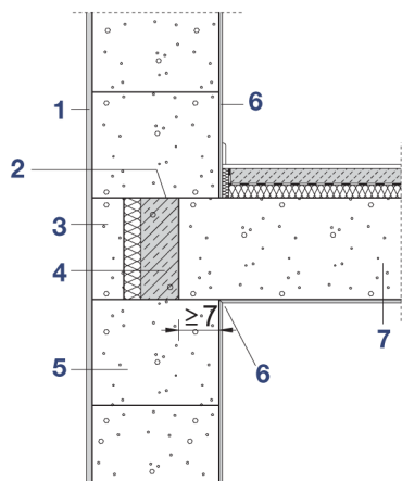
Figura 7a: Encuentro de un forjado de placas Ytong-Siporex con el muro exterior. Dintel de ventana prefabricado Ytong-Siporex.
