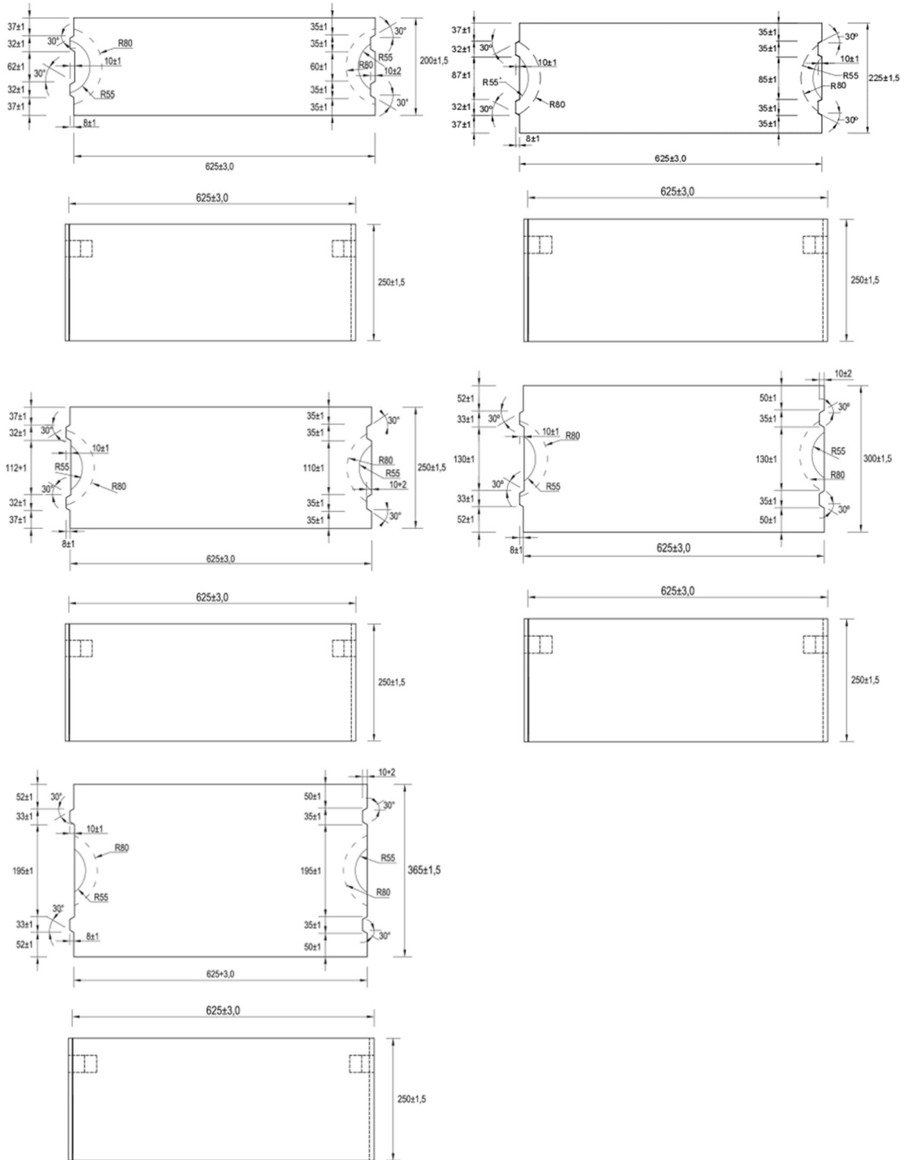
Figura 1: Geometría de los bloques TPE Ytong-Siporex (espesores 20, 22,5, 25, 30 y 36,5 cm).
