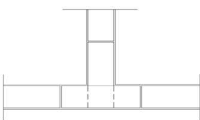
Figura 10: Unión en T de muros portantes Ytong-Siporex.
